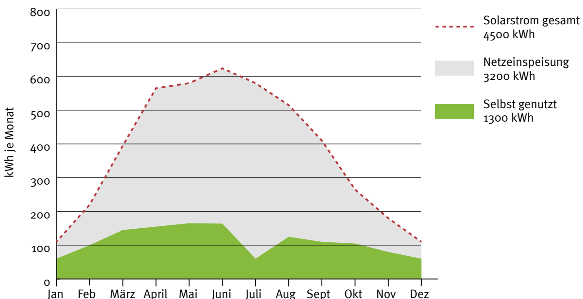
Beispielhafter Anteil des Eigenverbrauchs am selbst erzeugten Solarstrom
